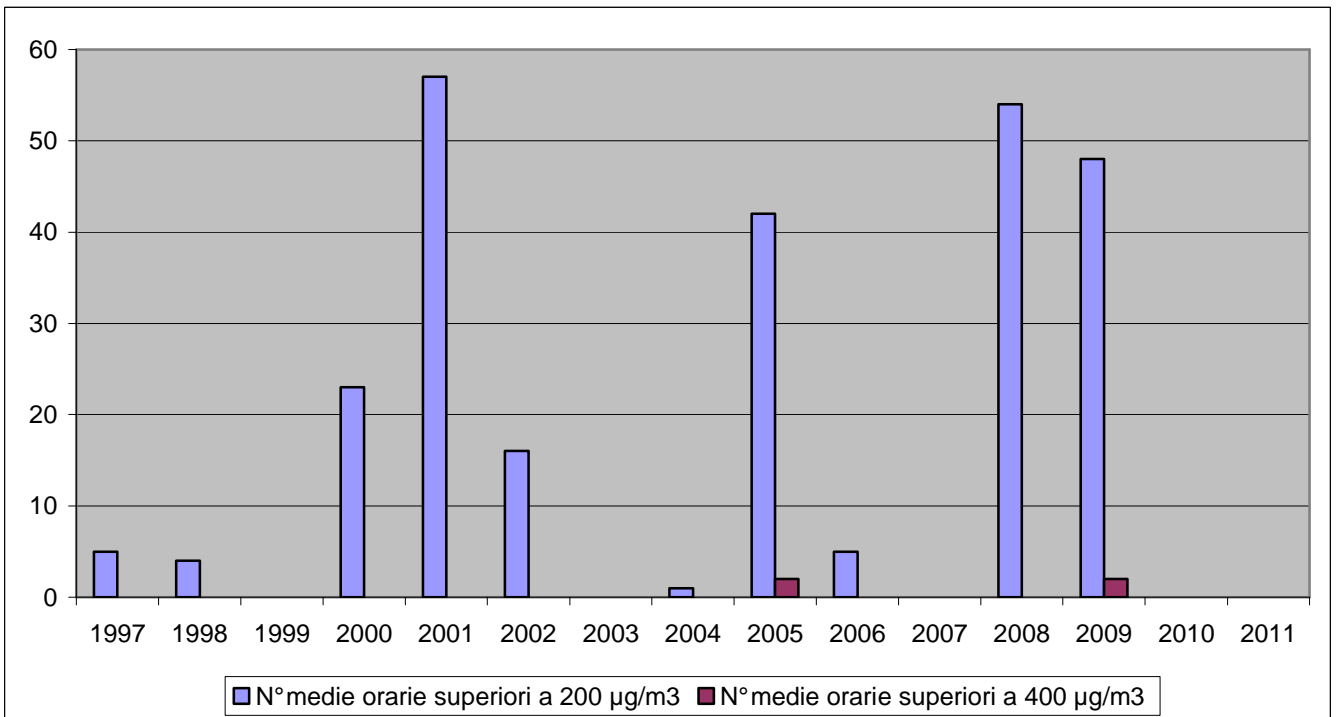
Piazza Plouves: Biossido di azoto nr. di medie orarie superiori a: Valore limite= 200 \mu\text{g}/\text{m}^3 Soglia di allarme = 400 \mu\text{g}/\text{m}^3
