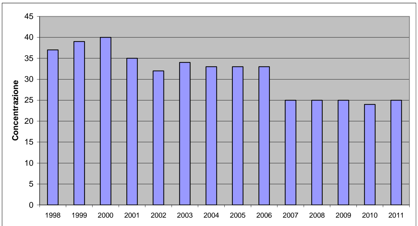
Piazza Plouves: medie annuali della concentrazione di PM 10 [ \mu\text{g}/\text{m}^3 ] (Polveri PM 10)
