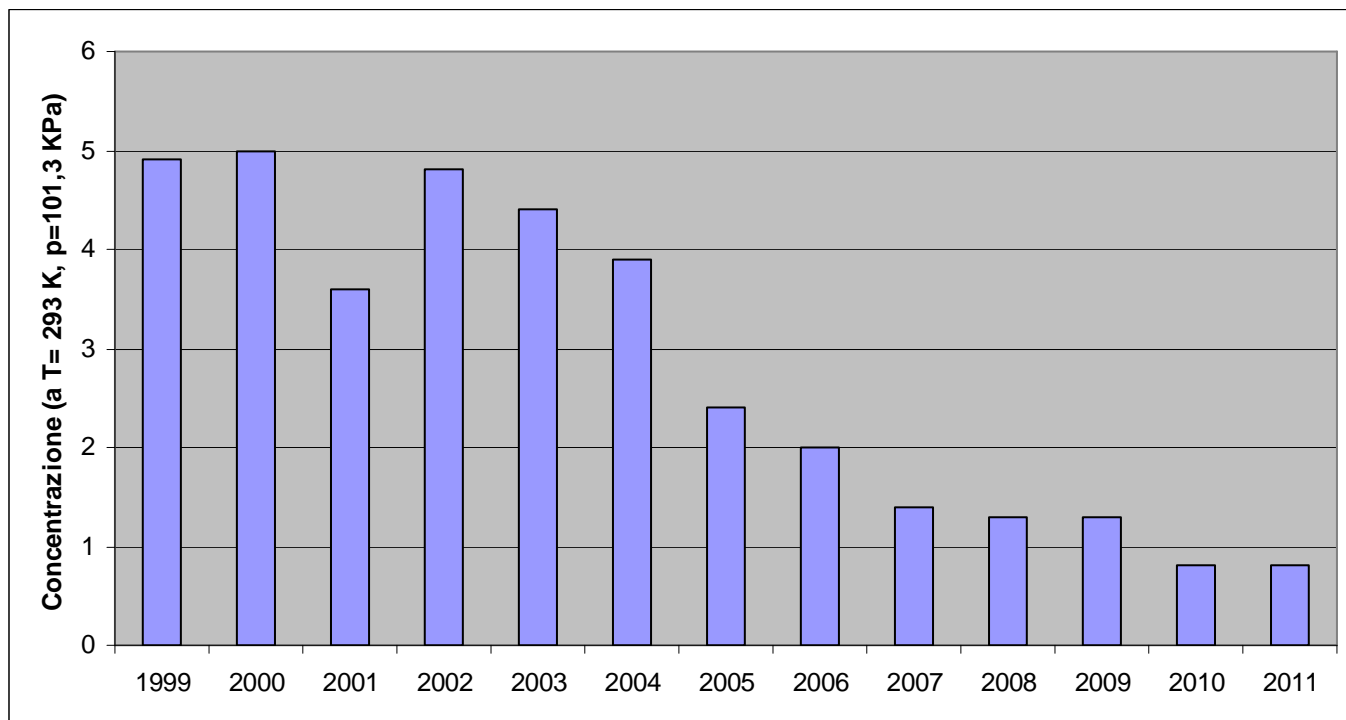
Piazza Plouves: medie annuali della concentrazione di C 6 H 6 [ \mu\text{g}/\text{m}^3 ] (Benzene)
