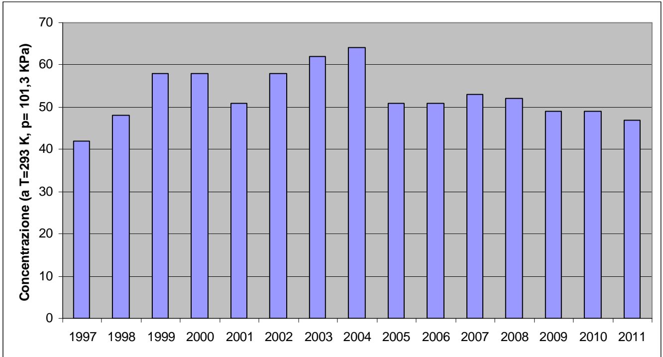
Medie annuali della concentrazione di O_3 [ \mu g/m^3 ] (Ozono)
