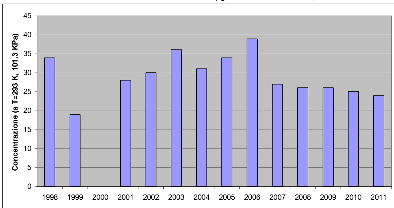
Medie annuali della concentrazione di \text{NO}_2 [ \mu\text{g}/\text{m}^3 ] (Biossido di Azoto)
