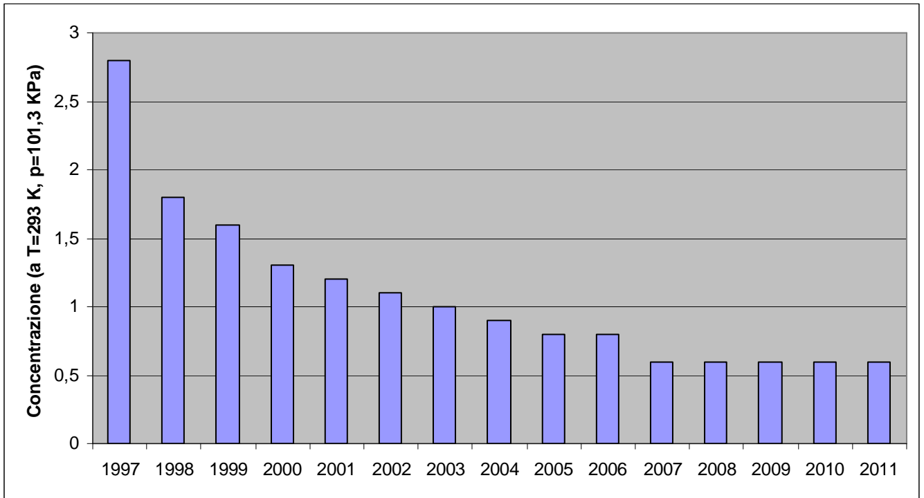
Piazza Plouves: medie annuali della concentrazione di CO [ \text{mg}/\text{m}^3 ] (Monossido di carbonio)
